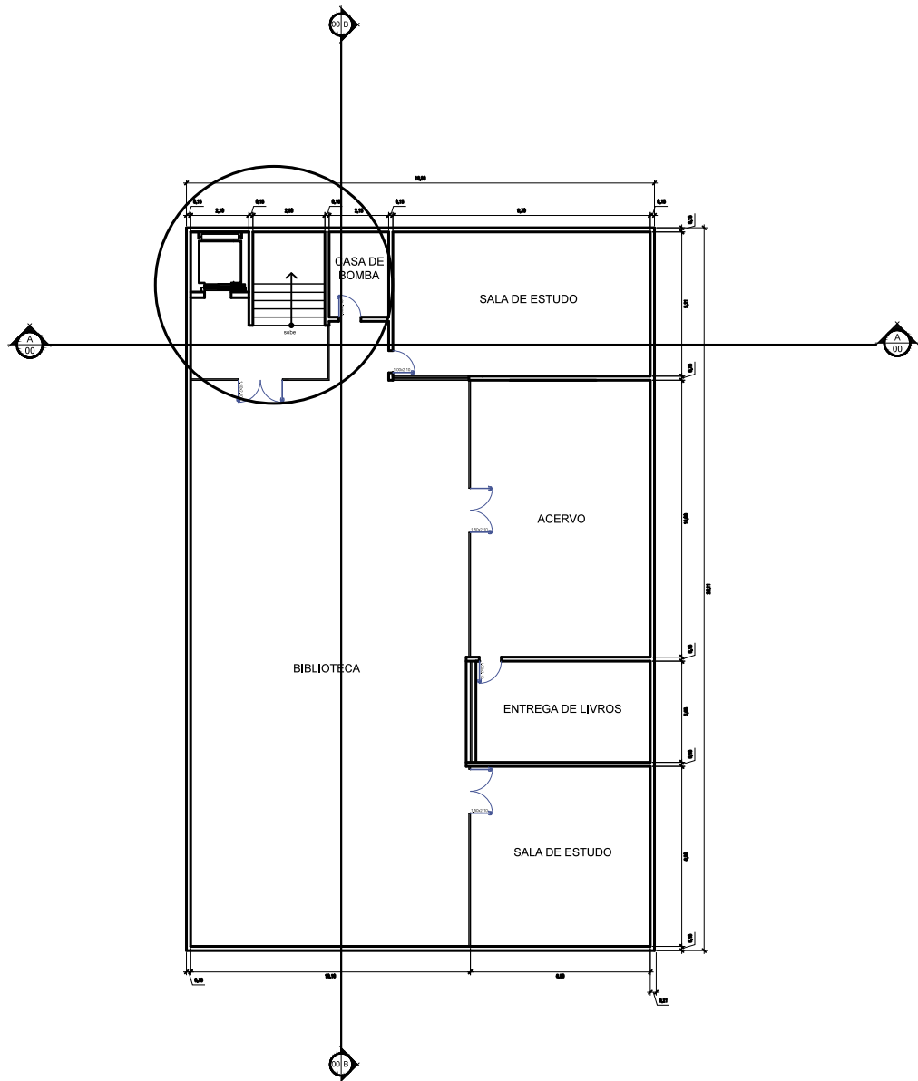
PLANTA BAIXA - SUBSOLO
