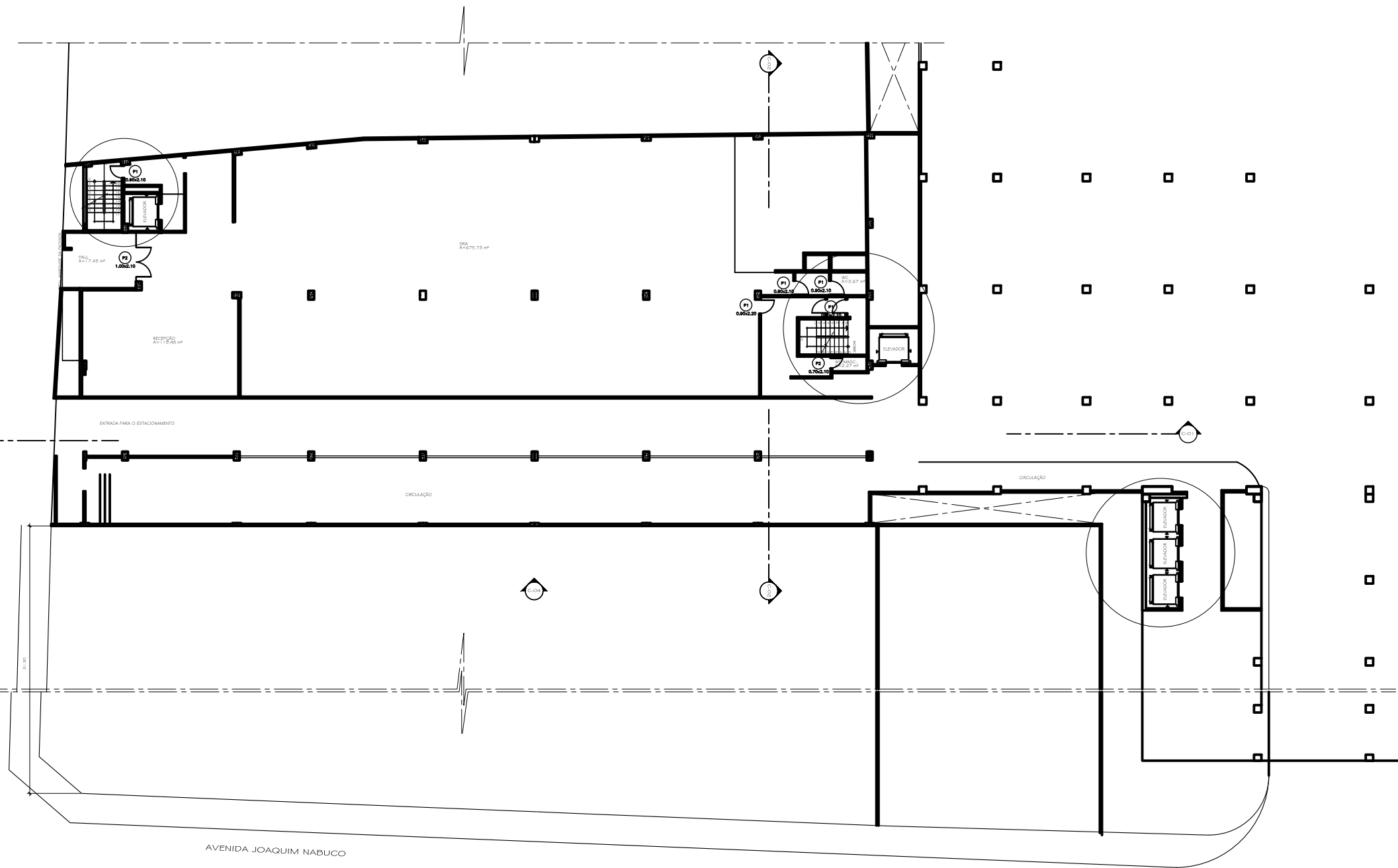
1/18 PLANTA BAIXA - TÉRREO NÍVEL -2.70 5000 - 1:100 ÁREA DO PAV. = 1.490,00 M 2
